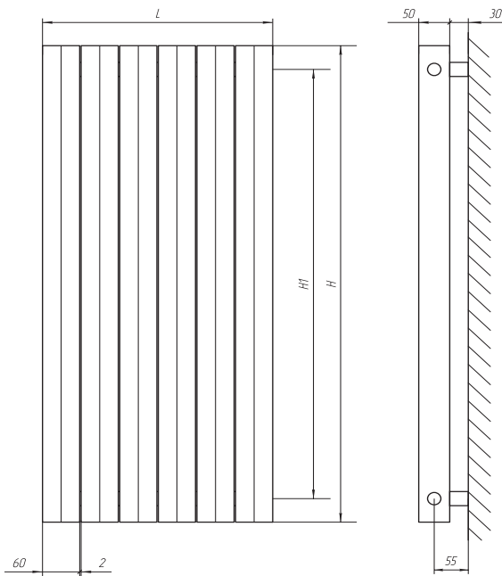
Боковое подключение
