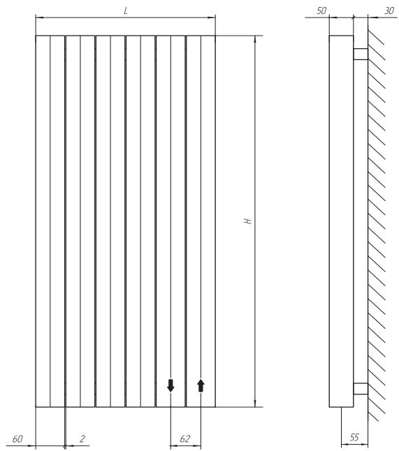
Нижнее подключение
