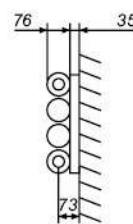
Нижнее подключение
